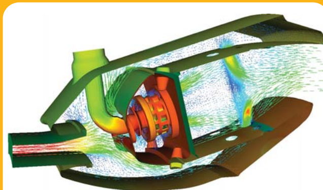
Calcul de combustion dans un moteur d'avion (Snecma Groupe Safran)
